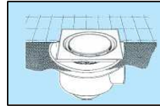
AD-CALDERETA 100 TELA ASFALTICA AD-CALDERETA SIFON V 200 90 AD-CALDERETA SIFON V 150 75 AD-CALDERETA SIFON V 250 110
