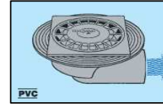
AD-CALDERETA SIFON H 150 75 AD-CALDERETA SIFON H 200 90 AD-CALDERETA SIFON H 200 110 AD-CALDERETA SIFON H 250 110
