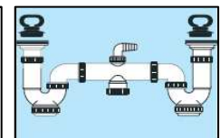
AD-SIFON forma P DOBLE T-7 AD-SIFON forma P DOBLE T-50
